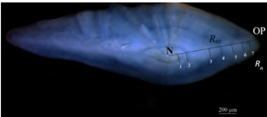
Figura 2.9 Bembrops heterurus : corte transversal de otólito sagitta mostrando o eixo de leitura e medição do raio da estrutura calcificada ( R_{ec} ) a partir do núcleo (N), os raios dos anéis de 1 a 7 ( R_n ) e o tipo de borda (OP = opaca)
