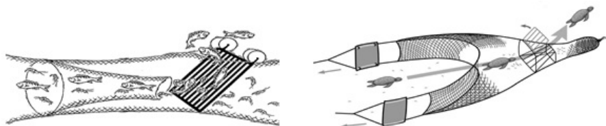
Figura 8.3 Dispositivos para o escape A) da fauna acompanhante em pesca de camarão, e B) de tartarugas-marinhas
