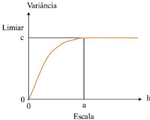
Figura 11.2 Comportamento ideal de um variograma estabelecido por Matheron, mostrando os parâmetros a (escala) e c (limiar).
