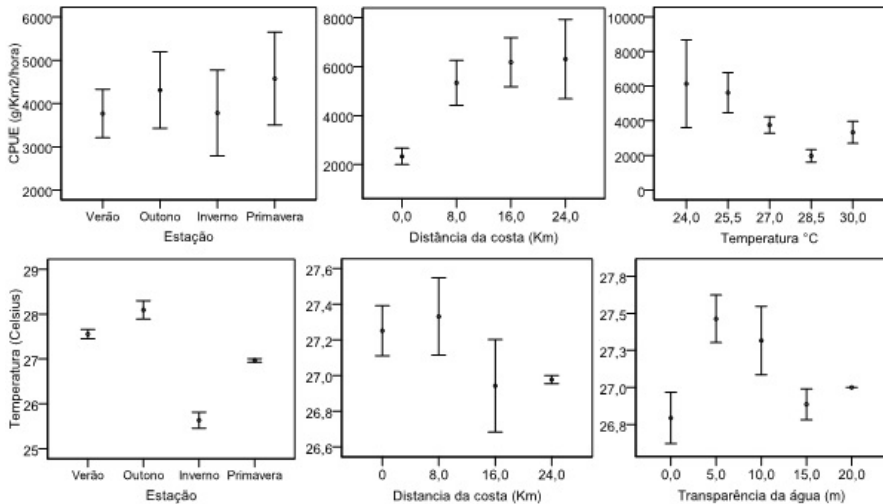
Figura 11.7 Índice de abundância relativo (CPUE) médio e erro padrão em relação à estação do ano (a), distância da costa (b) e temperatura da água (c). Temperatura média da água em relação a estação do ano (d), distância da costa (e) e transparência da água
